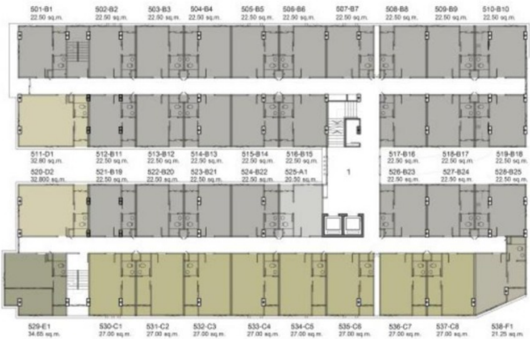
5 ЭТАЖ
